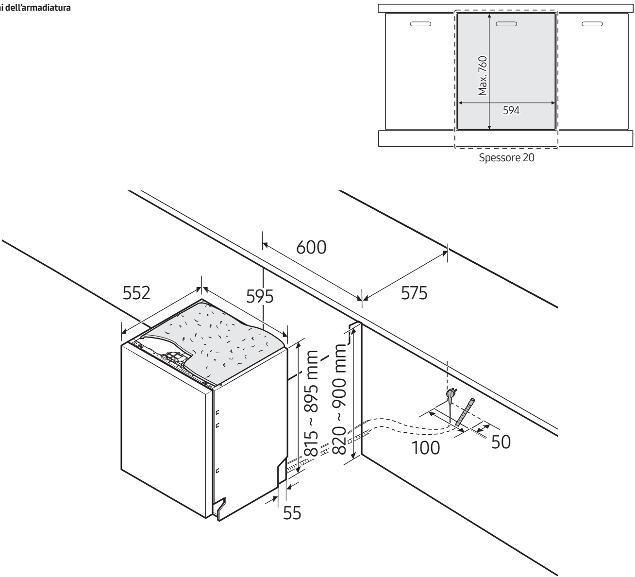
Dimensioni dell'armadiatura
