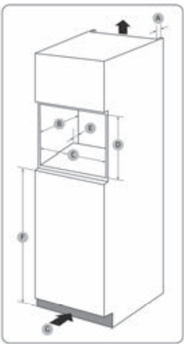
Dimensioni necessarie per l'installazione
