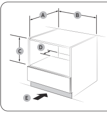
Struttura a incasso sotto lavello (mm)
